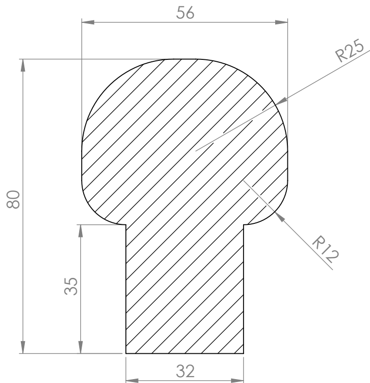
ŘEZ A-A
