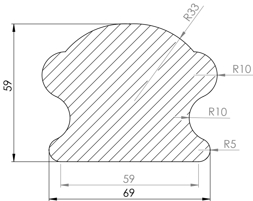
ŘEZ B-B
