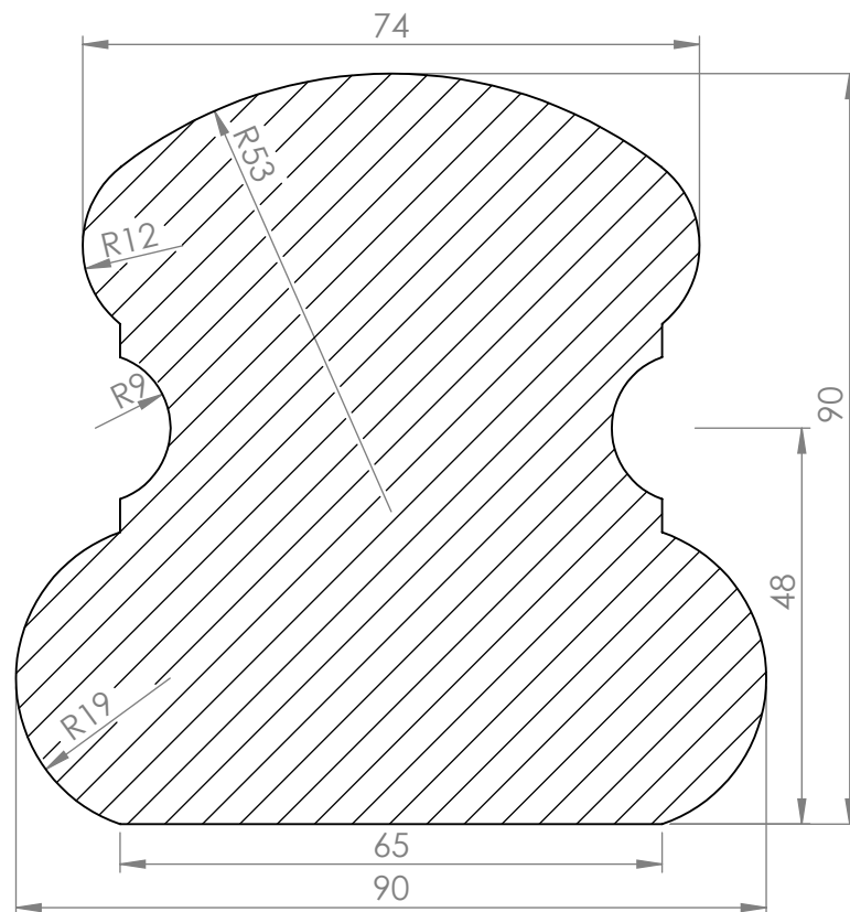
ŘEZ A-A
