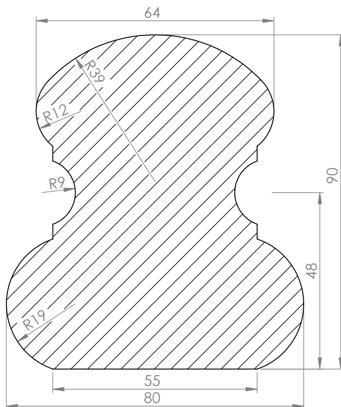
ŘEZ A-A
