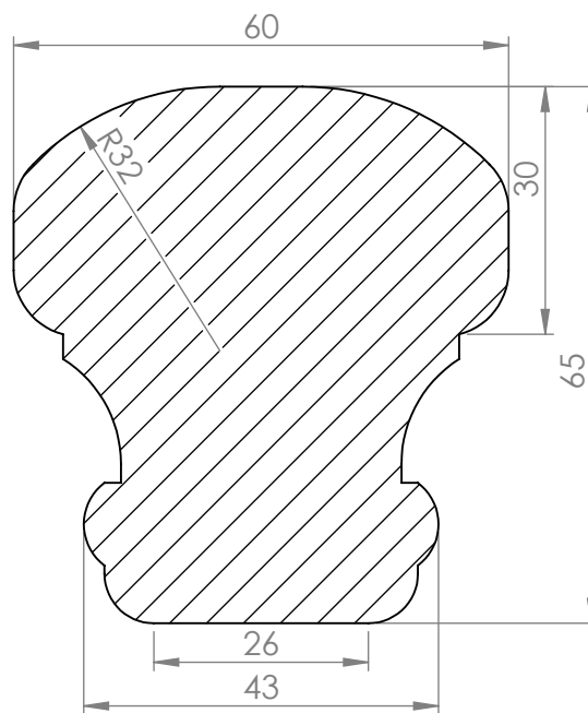
ŘEZ A-A
