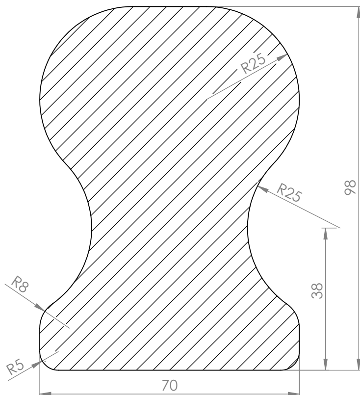
ŘEZ A-A
