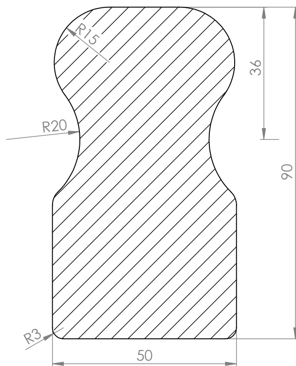
ŘEZ A-A
