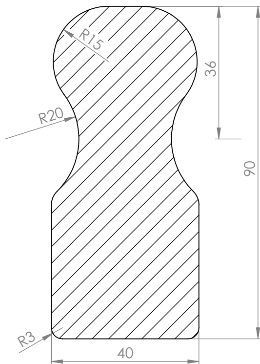
ŘEZ A-A
