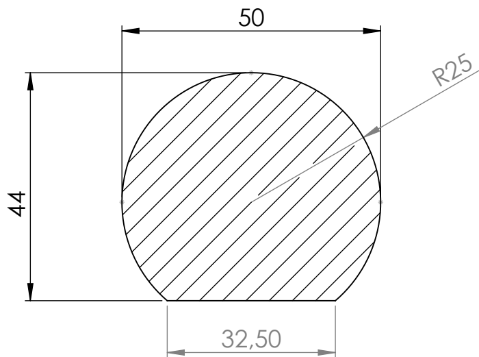
ŘEZ A-A
