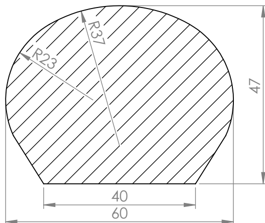
ŘEZ A-A
