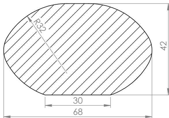
ŘEZ A-A
