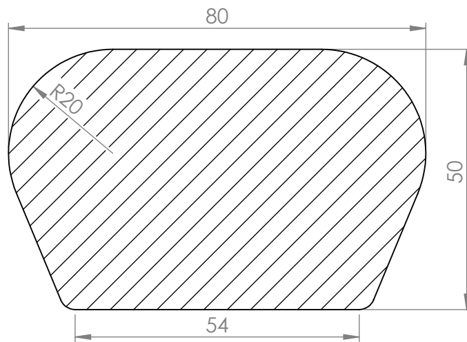
ŘEZ A-A
