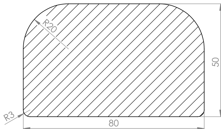
ŘEZ A-A
