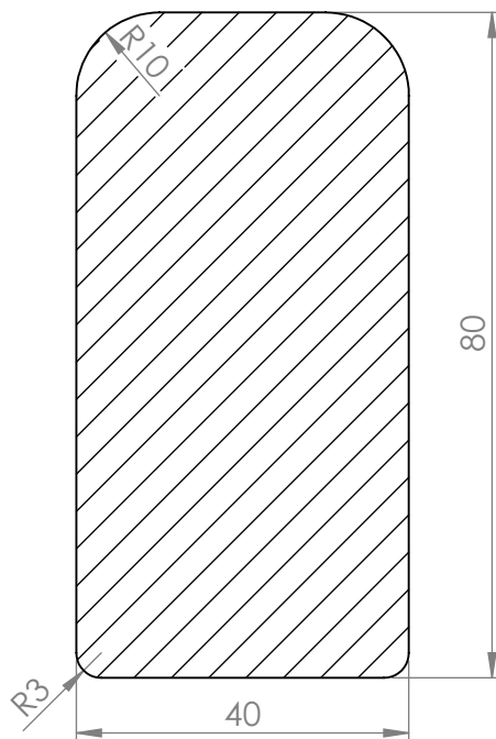
ŘEZ A-A
